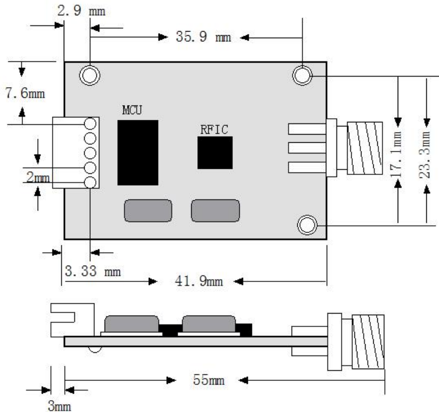
图5.1模块的尺寸结构图
