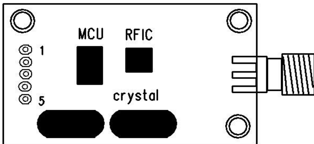
YL-100IL管脚排列图
