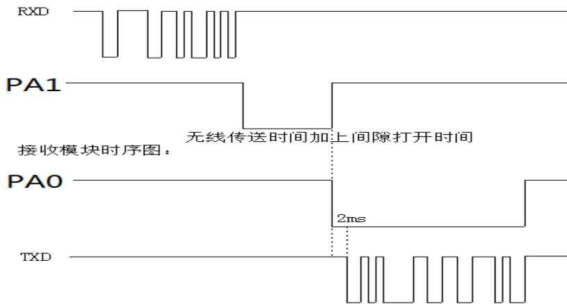
节点模式时序图
