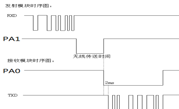
标准模式时序图
