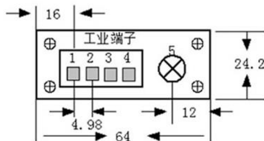
4pin 接线端子尺寸
