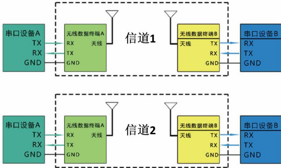
一对一通讯示意图，通过信道分组可以实现多条通讯线路同时进行
