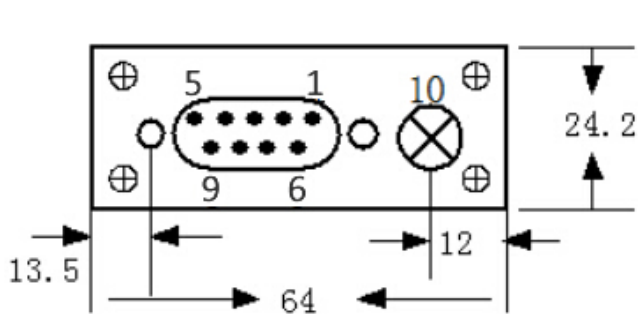
DB9 母头尺寸
