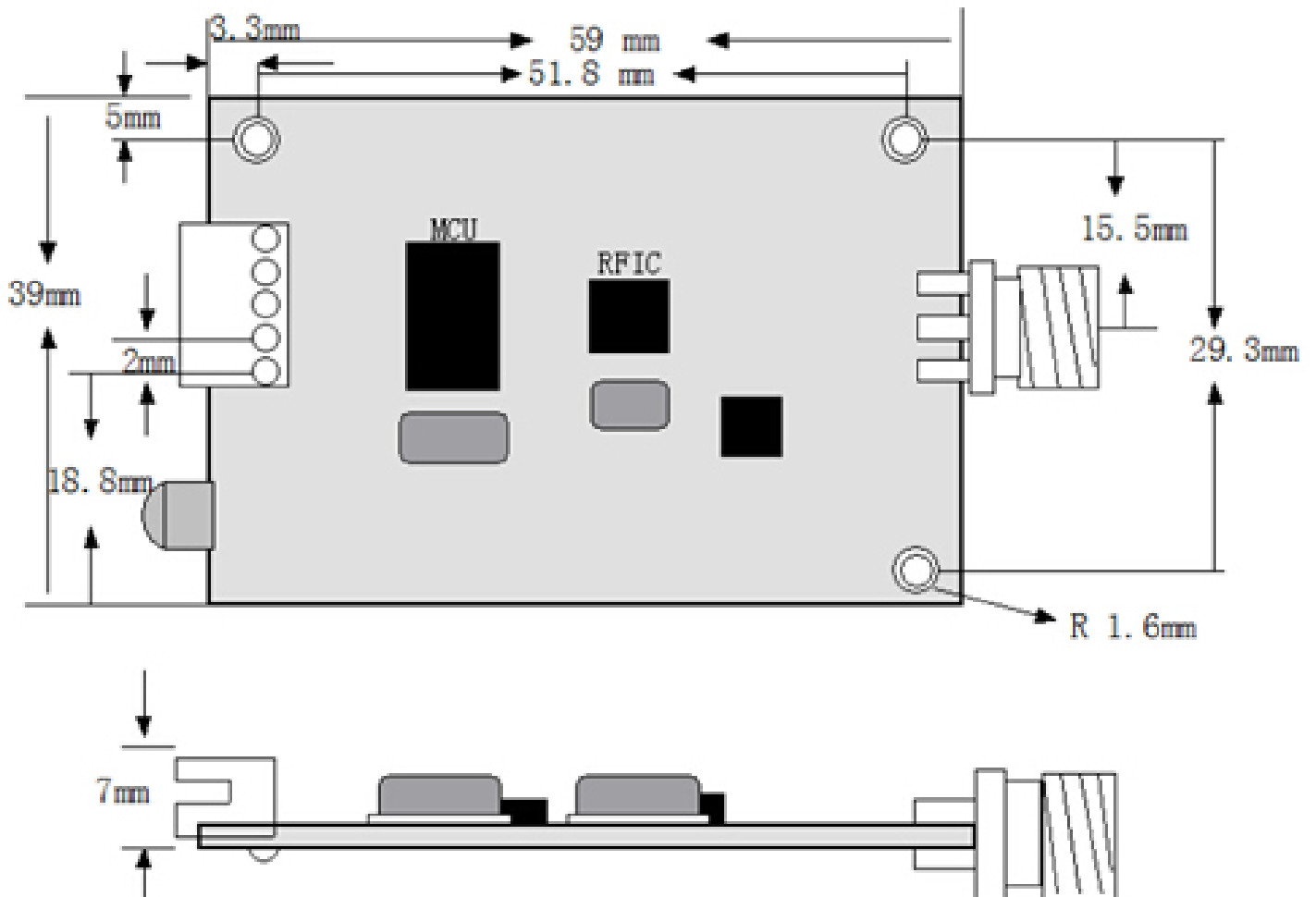
裸板模块尺寸结构
