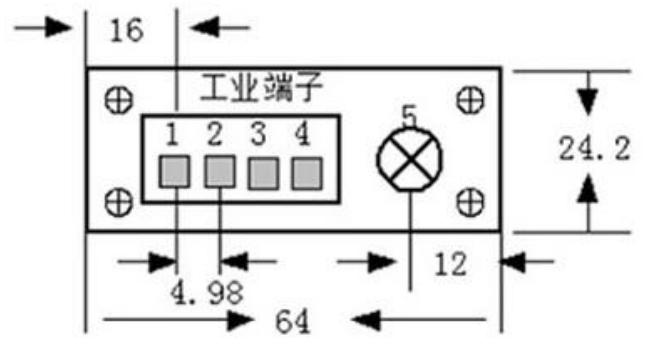
大银壳模块 4pin 端子封装规格
