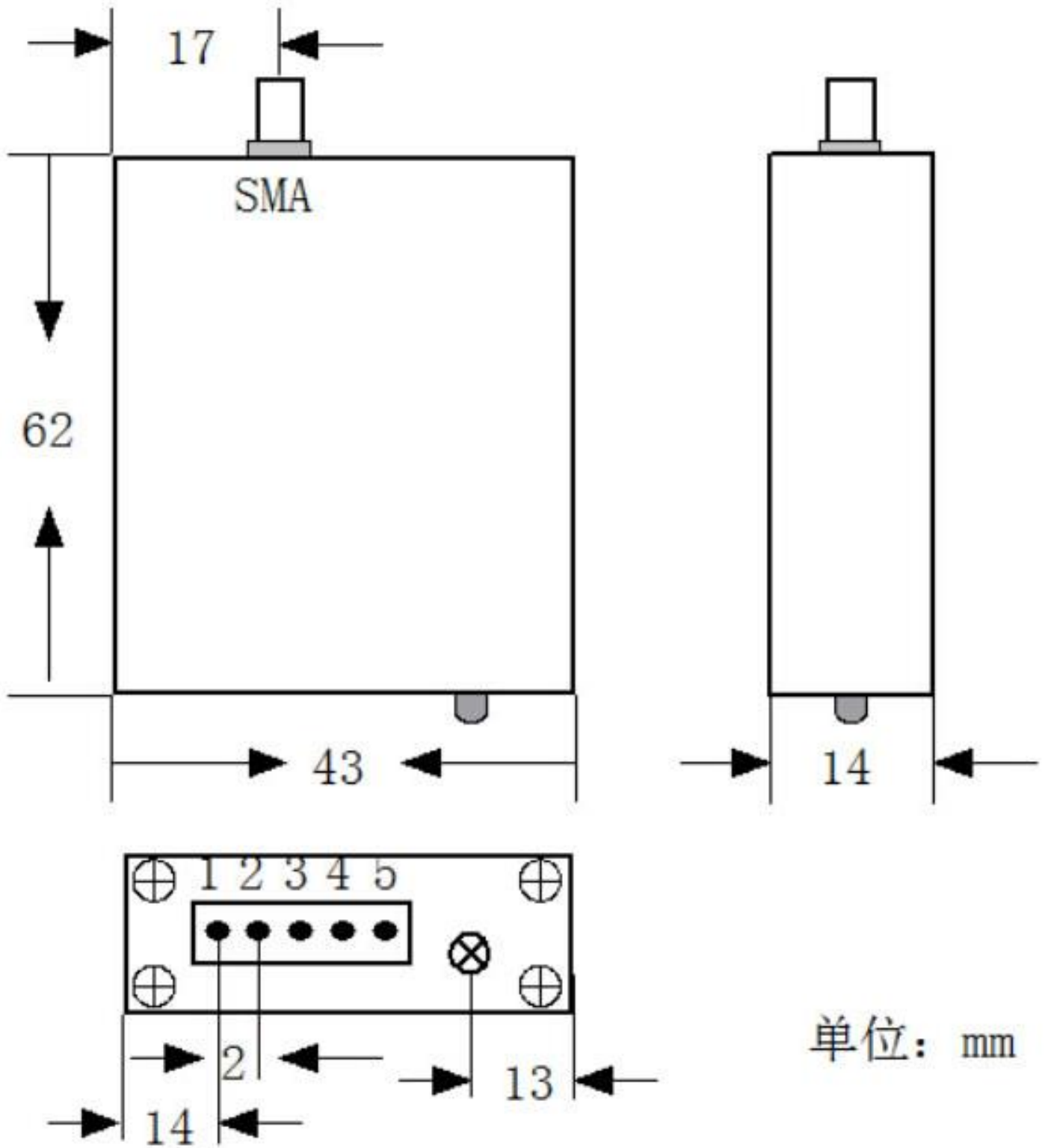
小黑壳模块尺寸结构图
