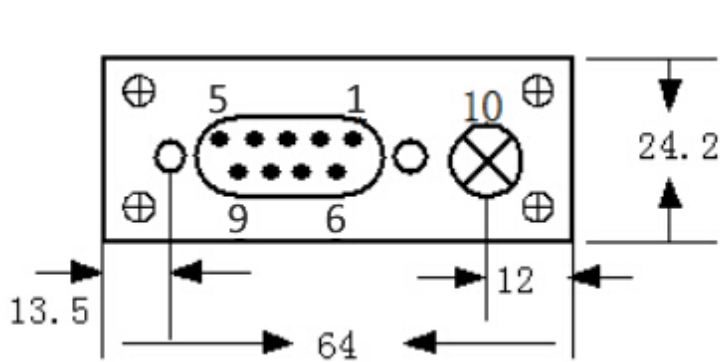
大银壳模块 DB9 母头封装规格
