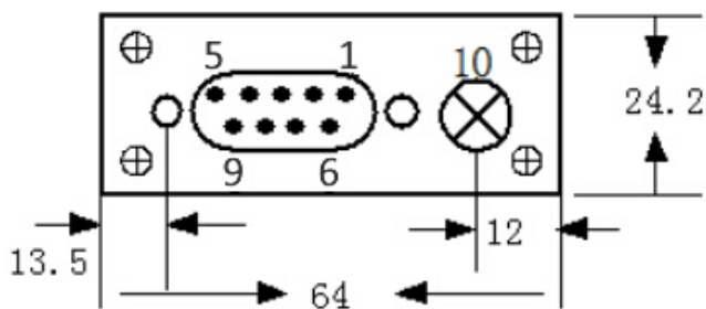
DB9 母头尺寸
