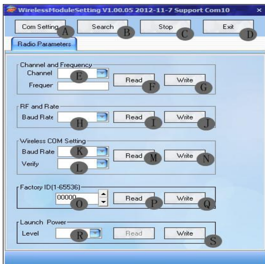
图 9.2 设置软件界面
