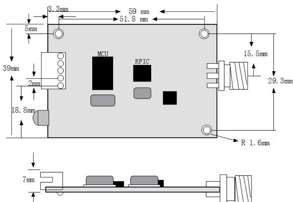
YL-500IL管脚排列图
