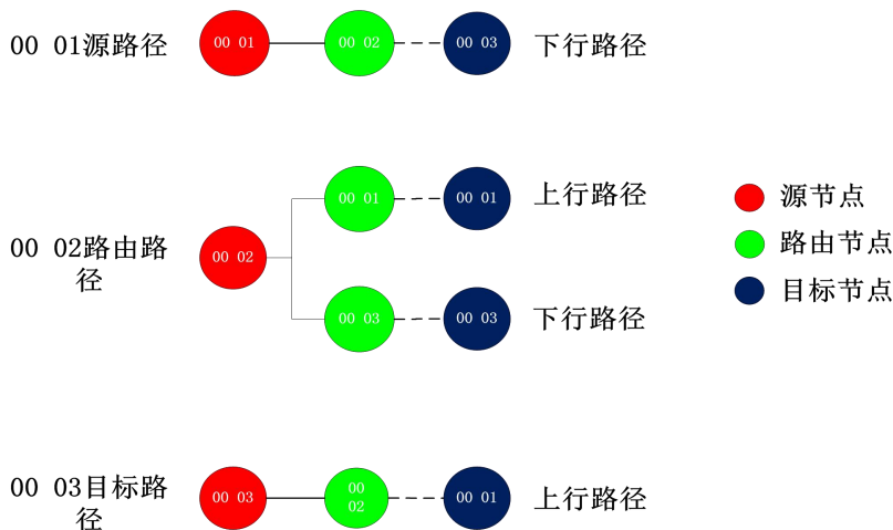
图 9.4.1 路由过程图
