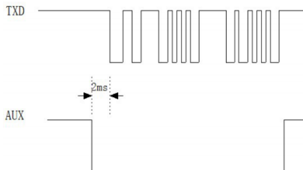
普通模式下 TXD 和 AUX 时序图
