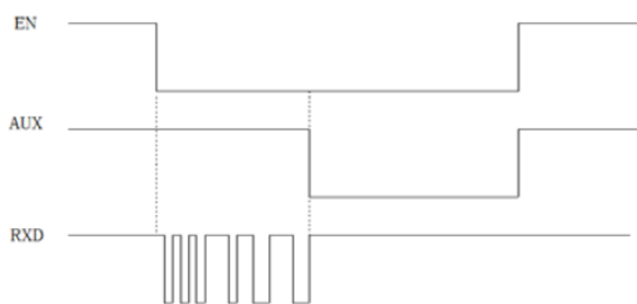
唤醒端时序图
