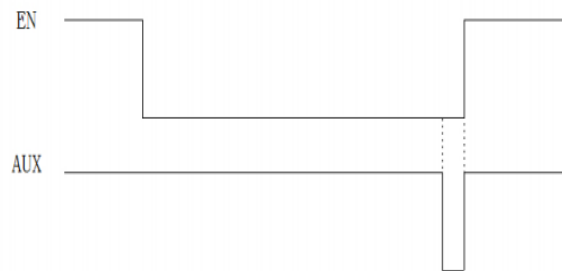
被唤醒端时序图
