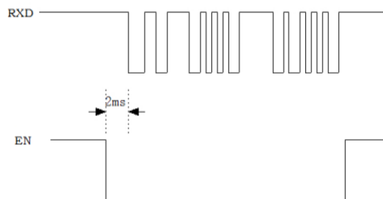
浅休眠模式下 RXD 和 EN 时序图
